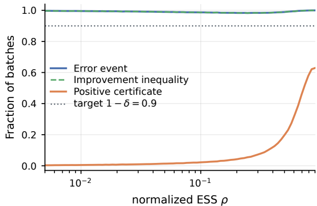
(d) One-step policy improvement
