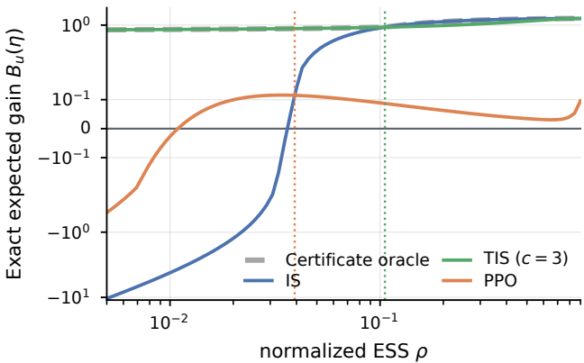
(d) One-step policy improvement
