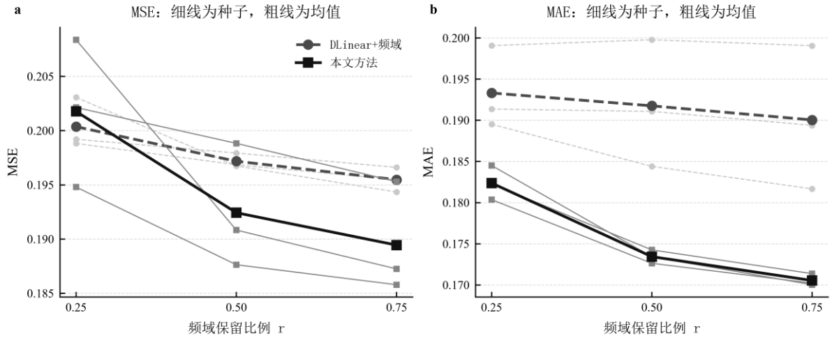
图 5 频率保留比例敏感性
