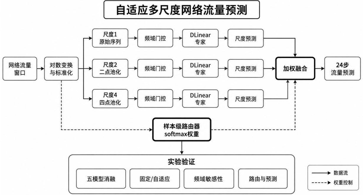
图 1 自适应多尺度预测框架
