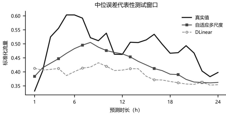
图6 代表性窗口预测结果
