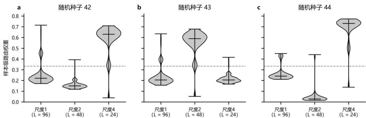
图 4 路由权重分布
