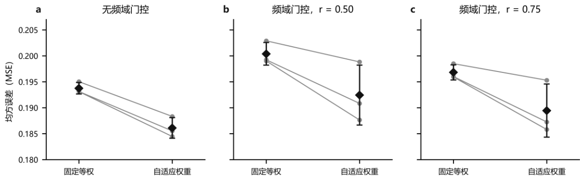
图 3 自适应权重消融结果
