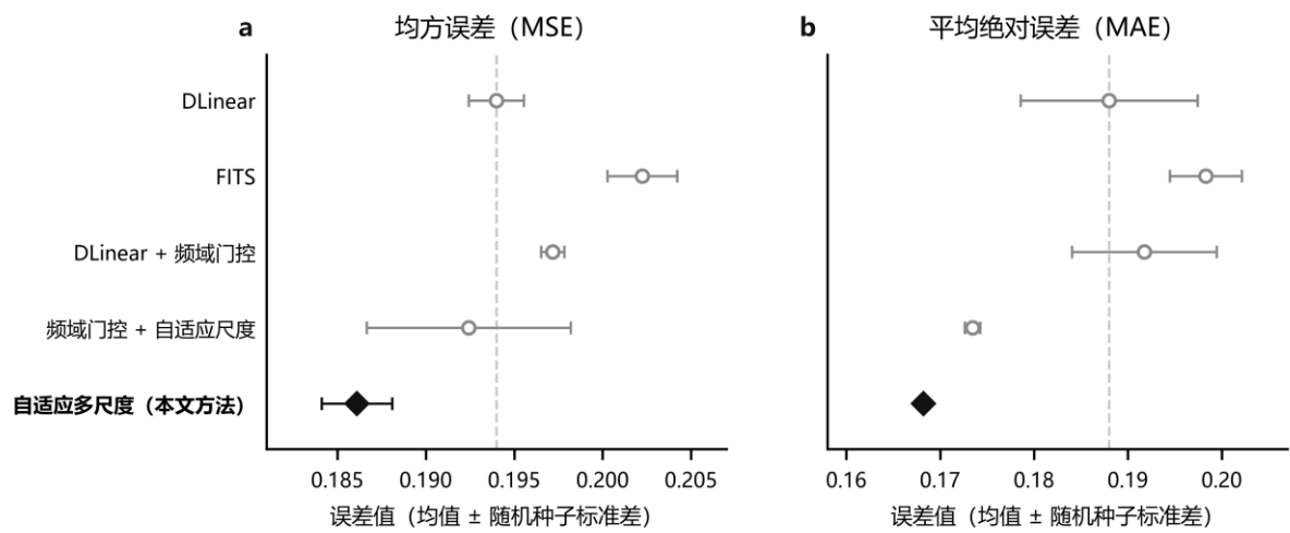
图 2 基础模型消融结果
