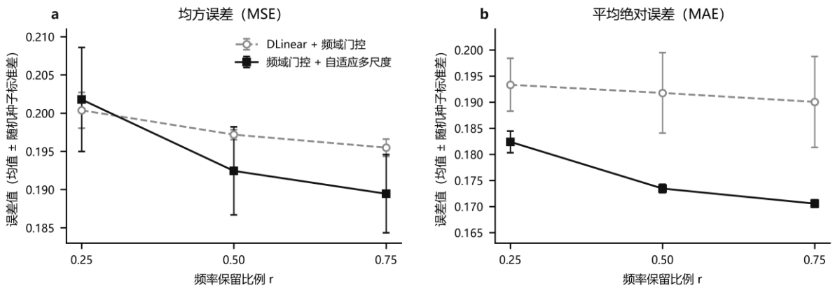
图 5 频率保留比例敏感性
