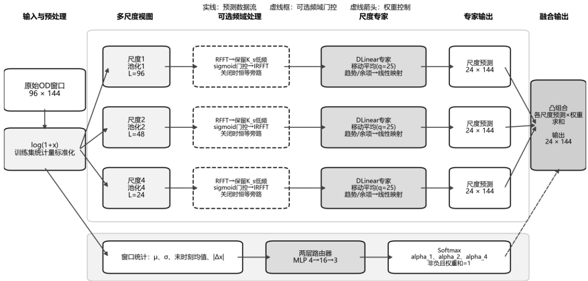
图 1 自适应多尺度预测框架
