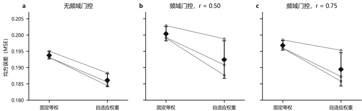
图 3 固定等权与自适应尺度权重的配对比较。细灰线连接同一随机种子，黑色菱形和误差线表示均值±样本标准差；a 为无频域，b、c 分别为 r=0.50 和 r=0.75。
