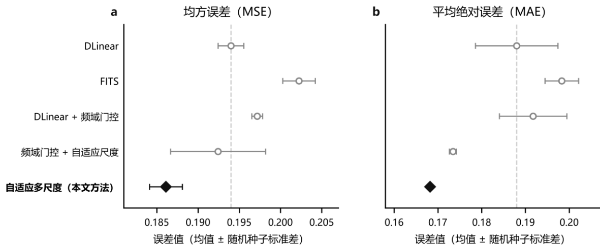
图 2 基础模型与组件消融。a 为测试集 MSE，b 为测试集 MAE；点表示三个随机种子的均值，误差线表示样本标准差，虚线为 DLinear 均值，黑色菱形为无频域自适应多尺度主模型。
