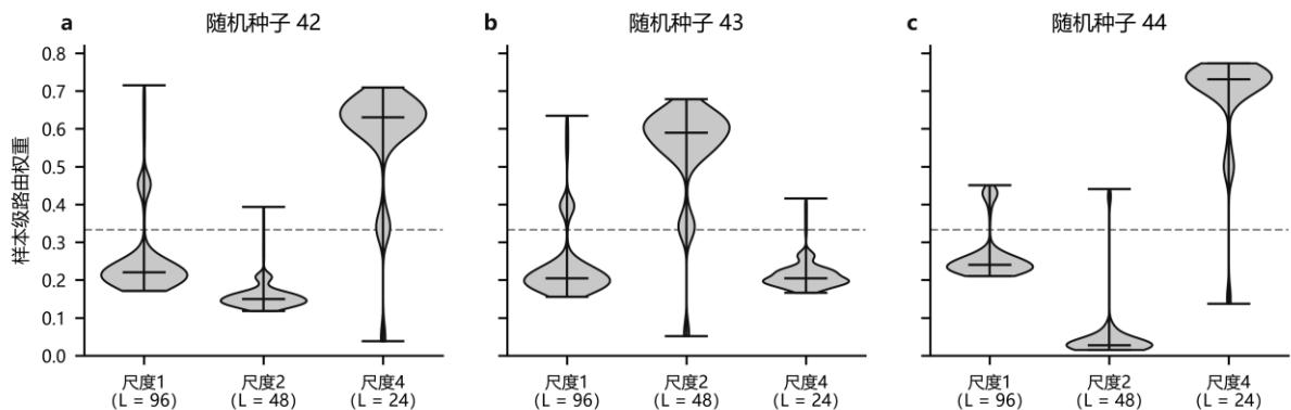
图 4 无频域自适应多尺度模型的样本级路由权重分布。a—c 对应种子 42、43 和 44；每幅图汇总 813 个测试窗口在尺度 1、2 和 4 上的 Softmax 权重，虚线为固定等权基准 1/3。
