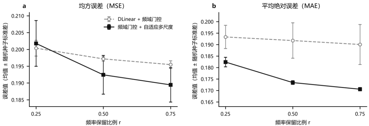
图 5 频率保留比例敏感性。a 为 MSE，b 为 MAE；虚线空心圆表示 DLinear+频域门控，实线实心方块表示频域门控+自适应多尺度，误差线为三个随机种子的样本标准差。
