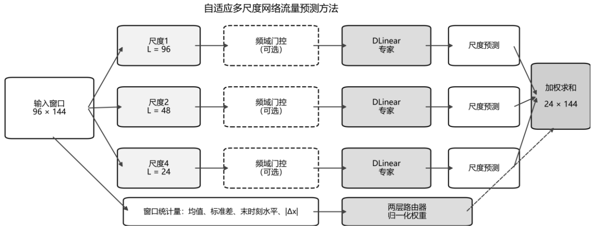
图 1 自适应多尺度网络流量预测方法结构。长度为 96、变量数为 144 的输入窗口经尺度 1、2 和 4 的非重叠平均池化，分别由 DLinear 专家产生未来 24 个时刻的预测；路由器依据四个窗口统计量生成样本级 Softmax 权重。虚线表示辅助频域分支。
