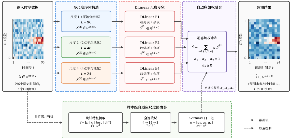
图 1 自适应多尺度网络流量预测方法框架
