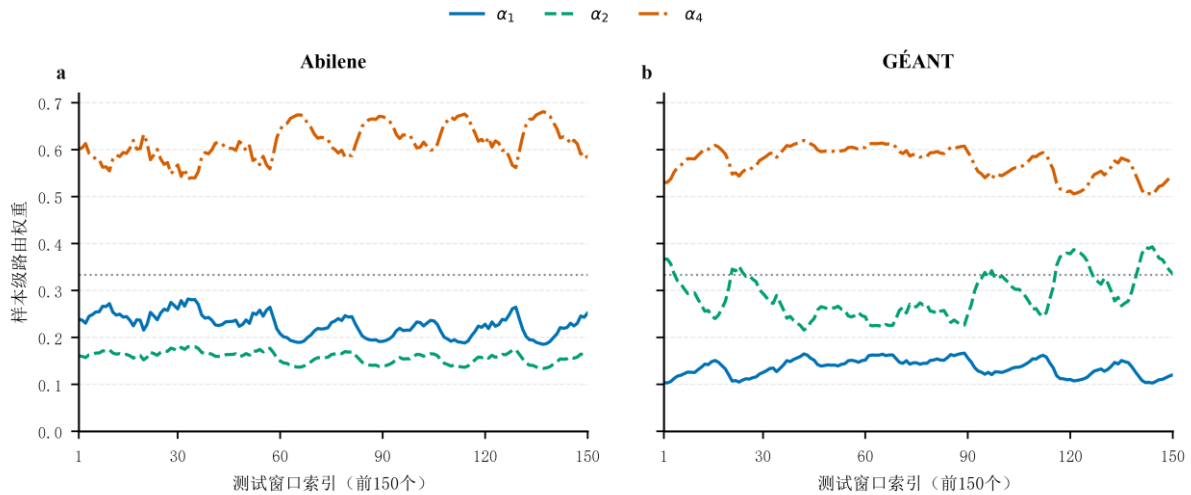
图 4 两数据集样本级路由权重变化（随机种子 42，灰色点线为等权基准 1/3）
