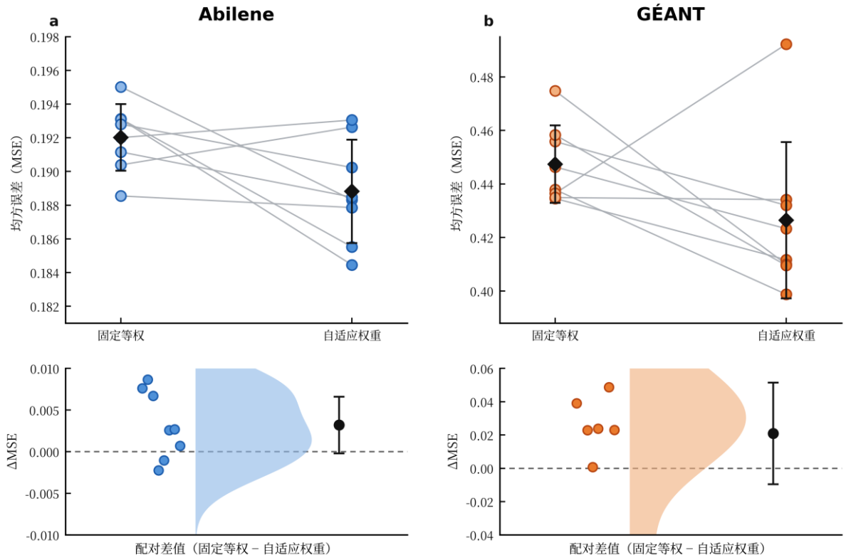
图 2 固定等权与自适应权重的八随机种子配对 MSE 及配对差值分布
