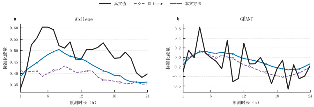
图 5 Abilene 与 GÉANT 代表性预测窗口的真实值与预测值对比（随机种子 42）
