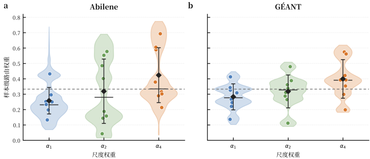
图 3 八随机种子下样本级自适应路由权重分布
