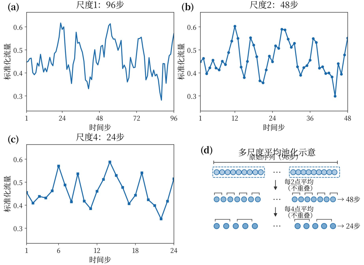
图 2 Abilene 单个 OD 变量的多尺度序列构造与平均池化示意
