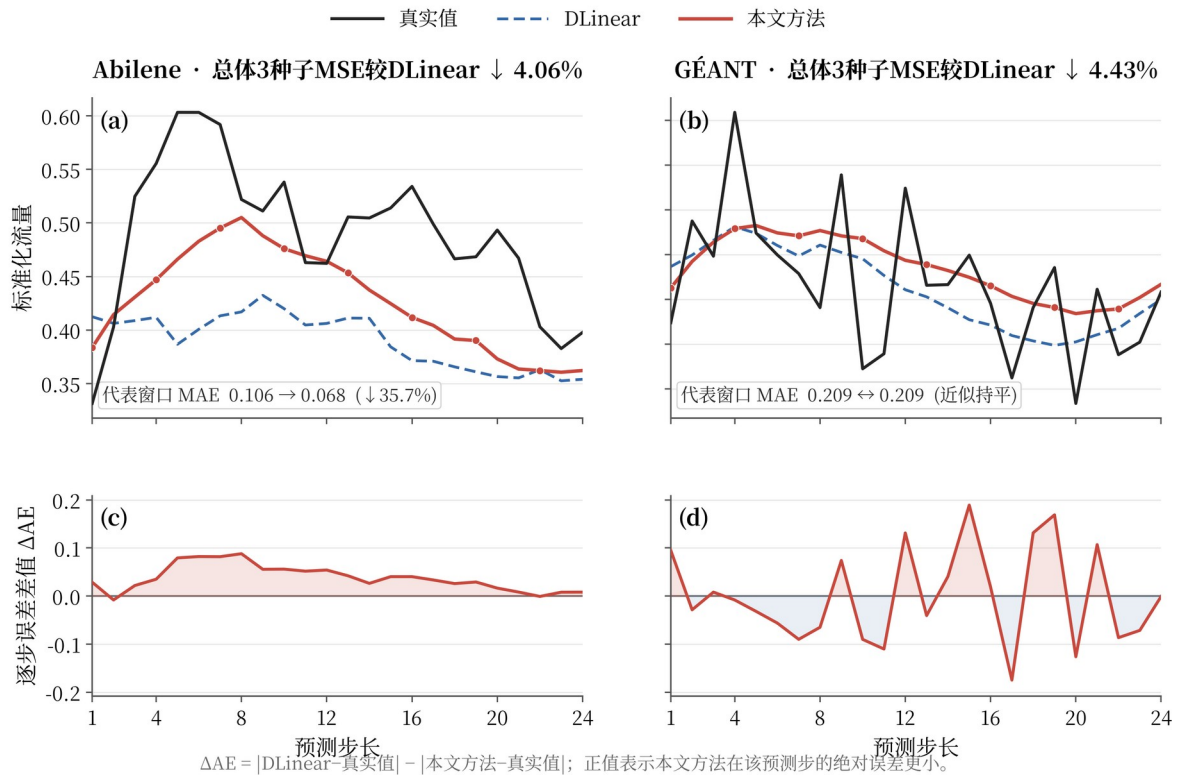
图4 Abilene 与 GÉANT 代表性测试窗口的 24 步预测及逐步误差差值
