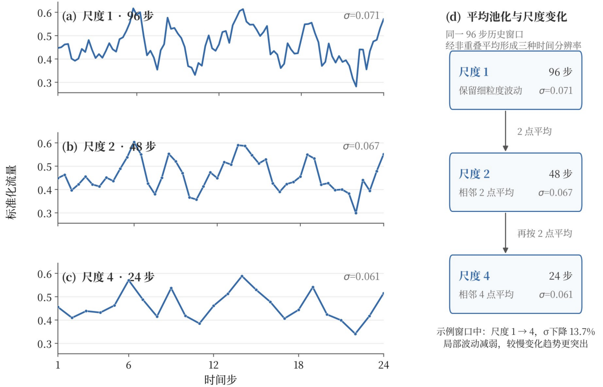
图 2 Abilene 单个 OD 变量的多尺度序列构造与平均池化示意
