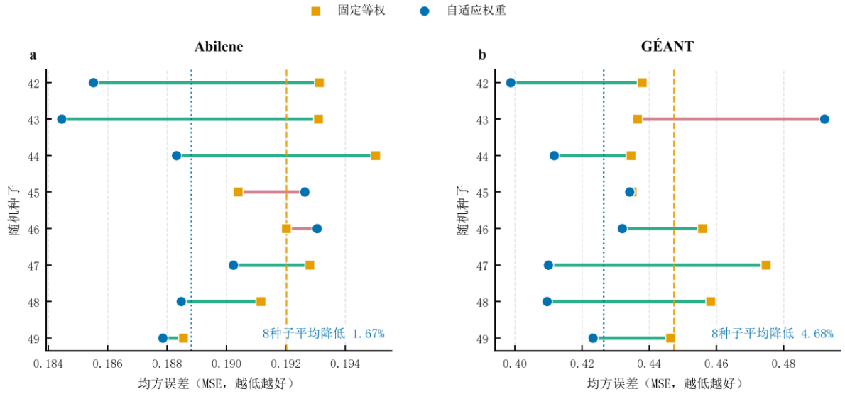
图2 固定等权与自适应权重的八随机种子配对 MSE（橙色方形与蓝色圆形分别表示固定等权和自适应权重；绿色连线表示误差降低，红色连线表示误差升高；竖向虚线和点线表示两模型 8 种子均值）
