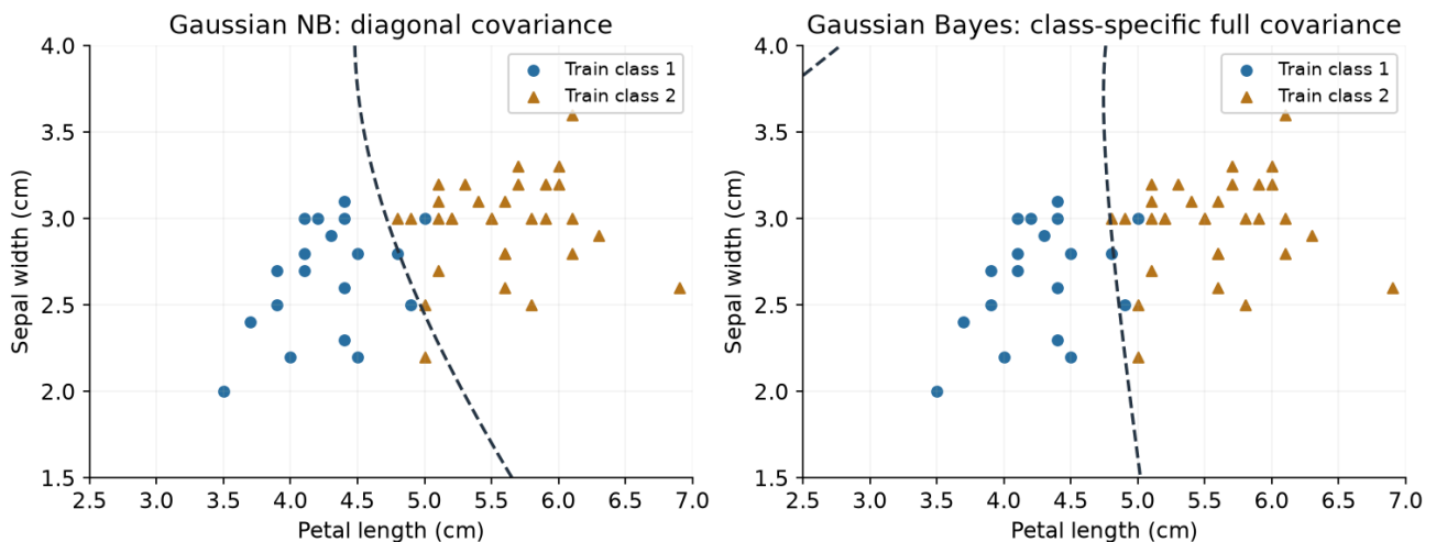
图：沿用原 B12 的50/50划分与种子4487，完整高斯保留原 numpy.cov 的 N_c-1 约定；点仅显示训练记录，虚线为两类后验相等处。测试集比较见下文；图中显示的是训练记录。
