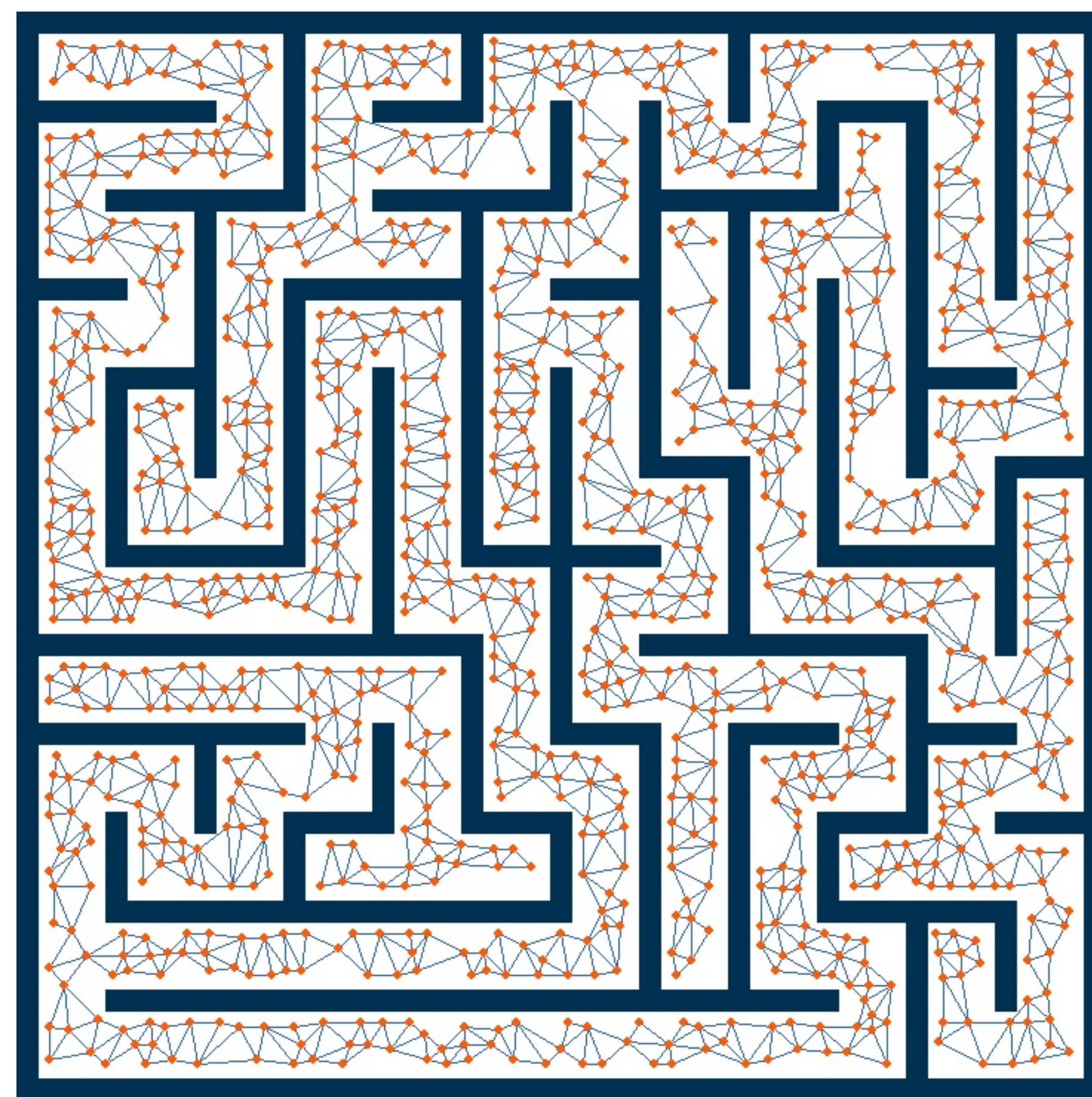
(d) GSRM Maze
