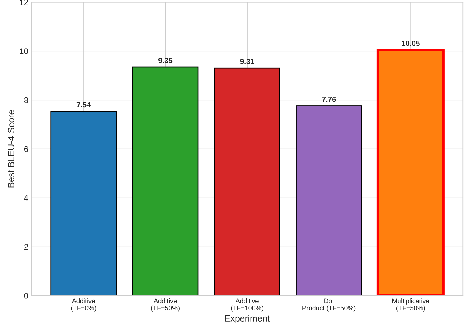
(d) Best BLEU-4 Score Comparison
