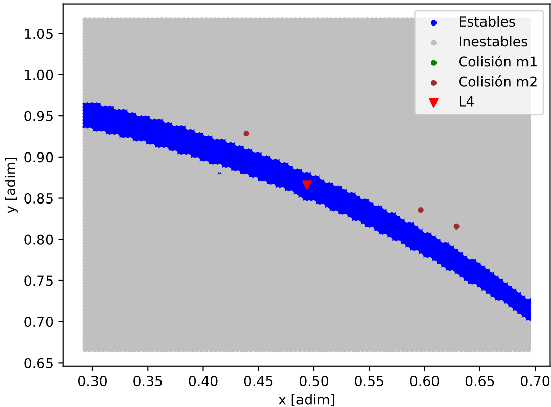
Mapa de estabilidad - HAT-P-2
