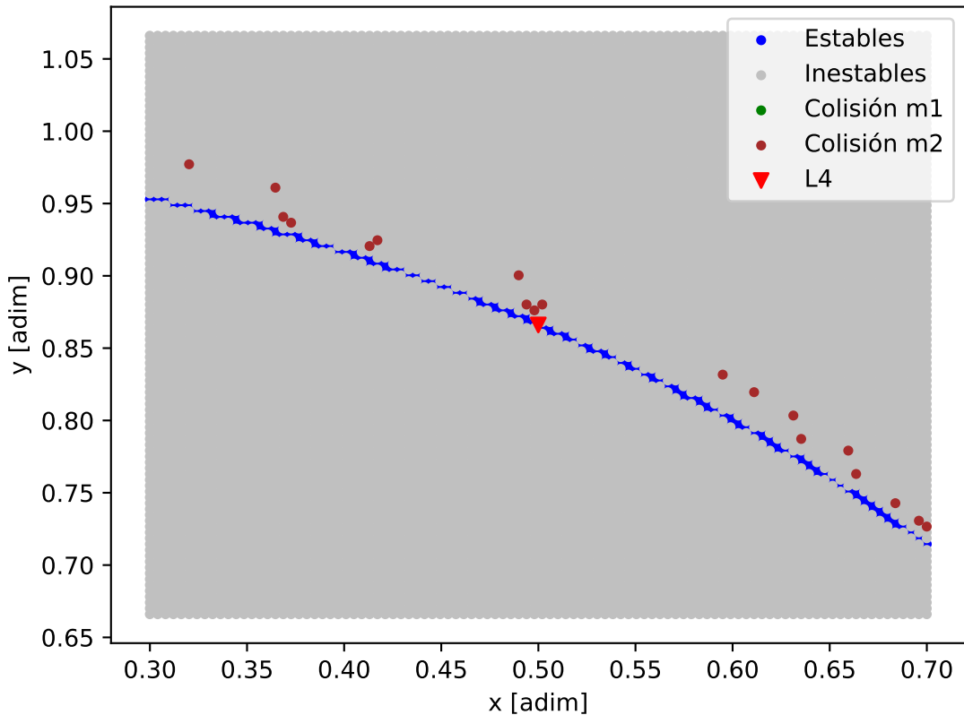
Mapa de estabilidad - HD_106315
