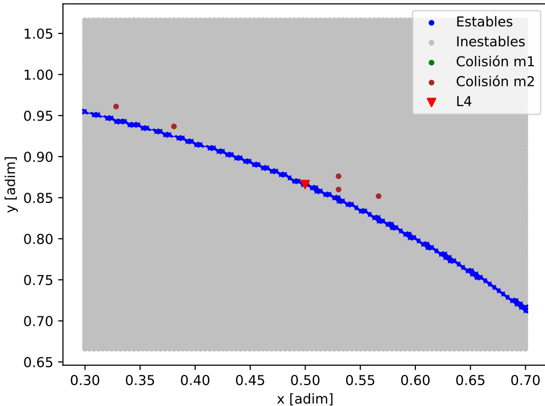
Mapa de estabilidad - Kepler-117
