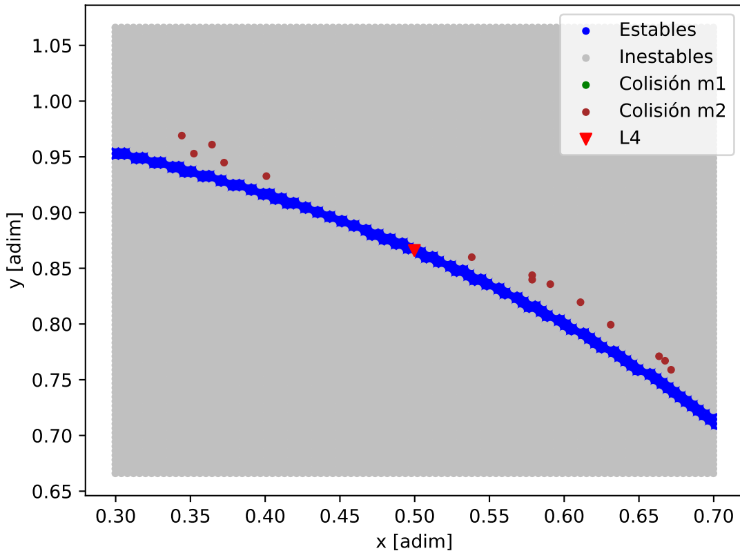
Mapa de estabilidad - TOI-1338_A
