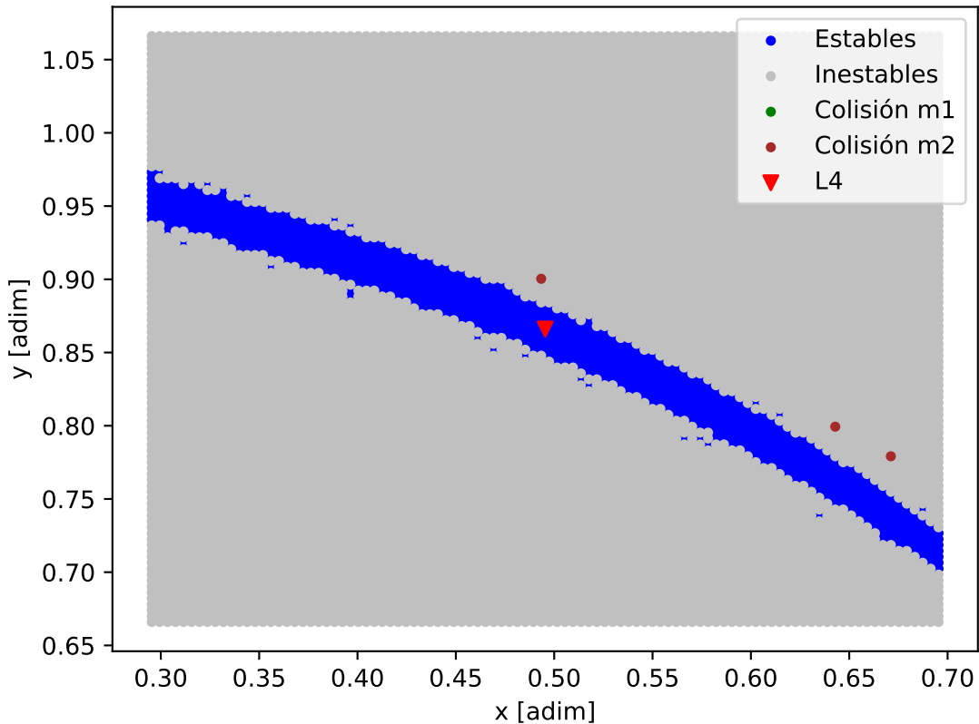
Mapa de estabilidad - TOI-4562
