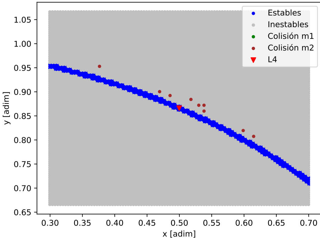
Mapa de estabilidad - WASP-94_A
