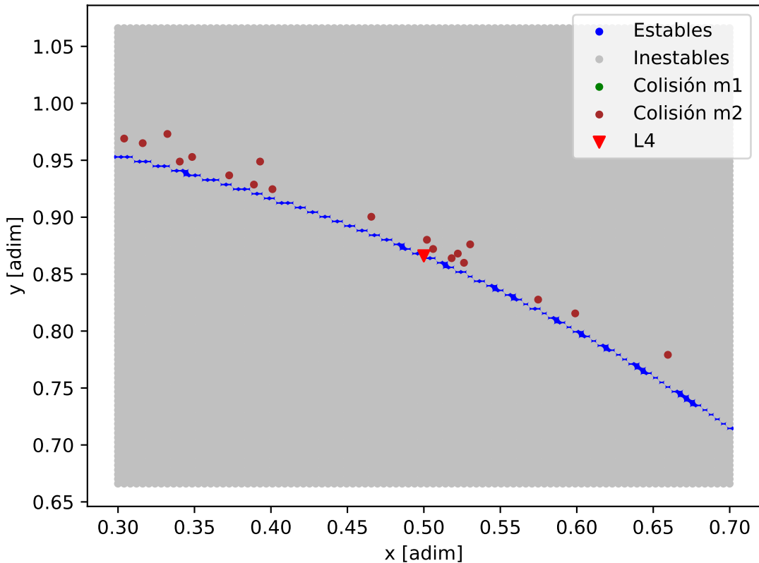
Mapa de estabilidad - 55_Cnc
