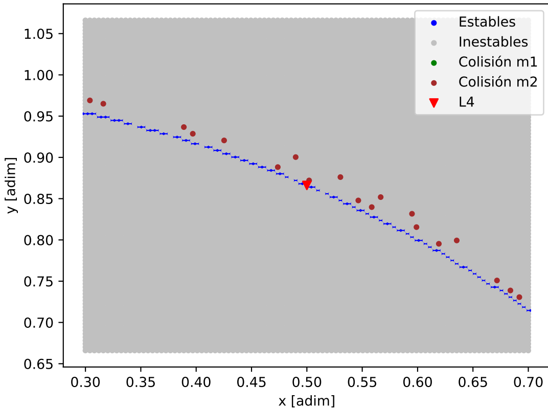
Mapa de estabilidad - CoRoT-7
