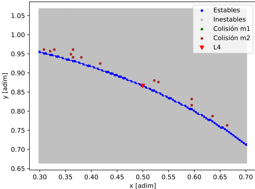
Mapa de estabilidad - HD_107148
