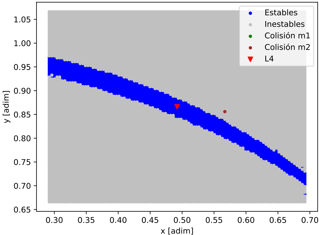
Mapa de estabilidad - HD_111232
