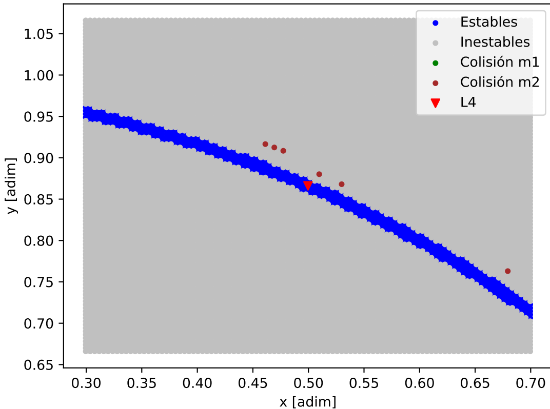
Mapa de estabilidad - HD_133131_A
