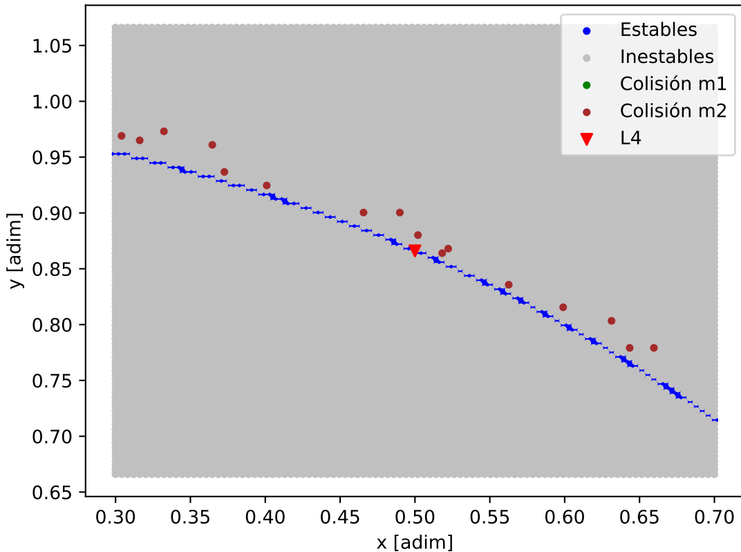
Mapa de estabilidad - HD_152843
