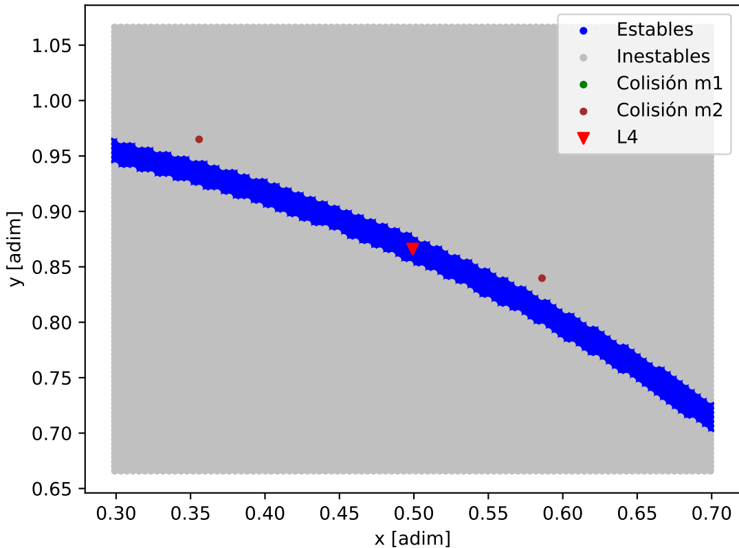
Mapa de estabilidad - HD_153358
