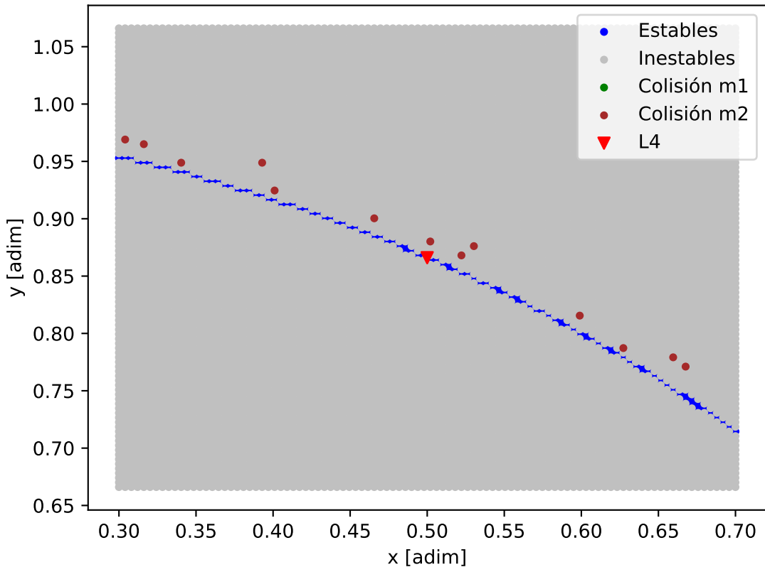
Mapa de estabilidad - HD_155918
