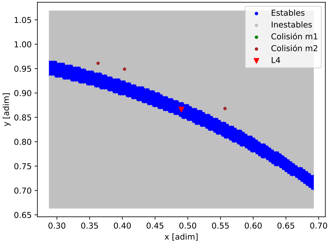
Mapa de estabilidad - HD_156279
