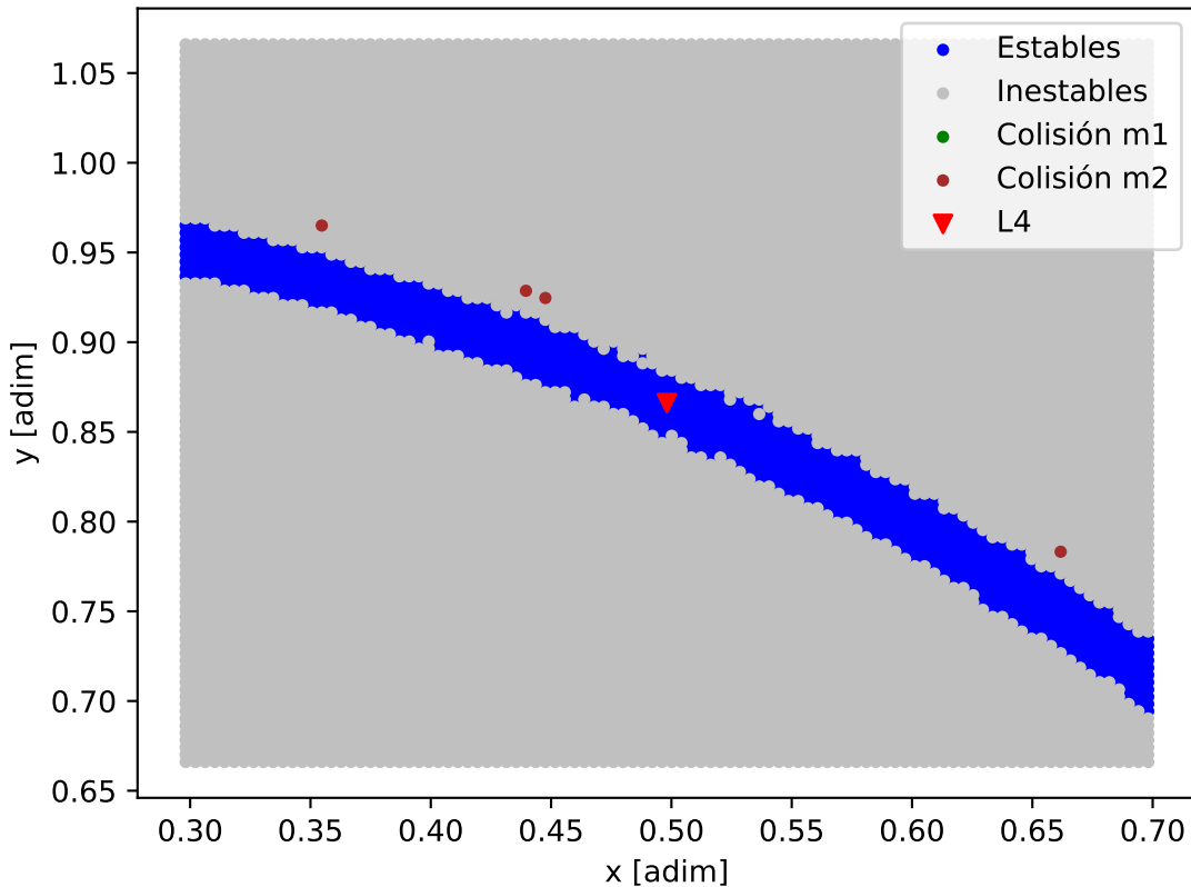
Mapa de estabilidad - HD_163607
