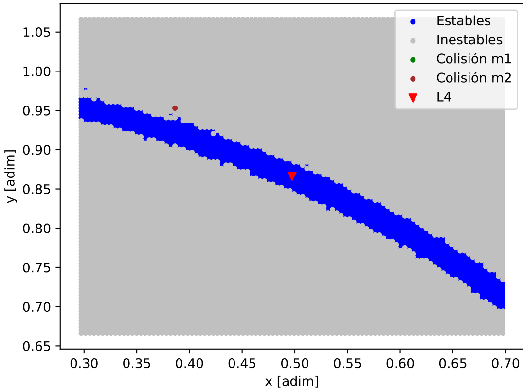
Mapa de estabilidad - HD_187123
