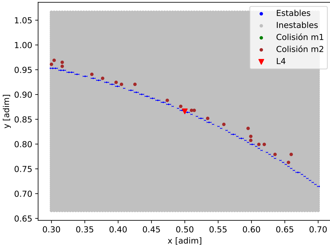
Mapa de estabilidad - HD_191939
