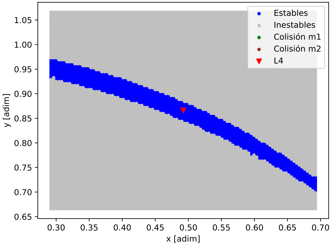
Mapa de estabilidad - HD_43197
