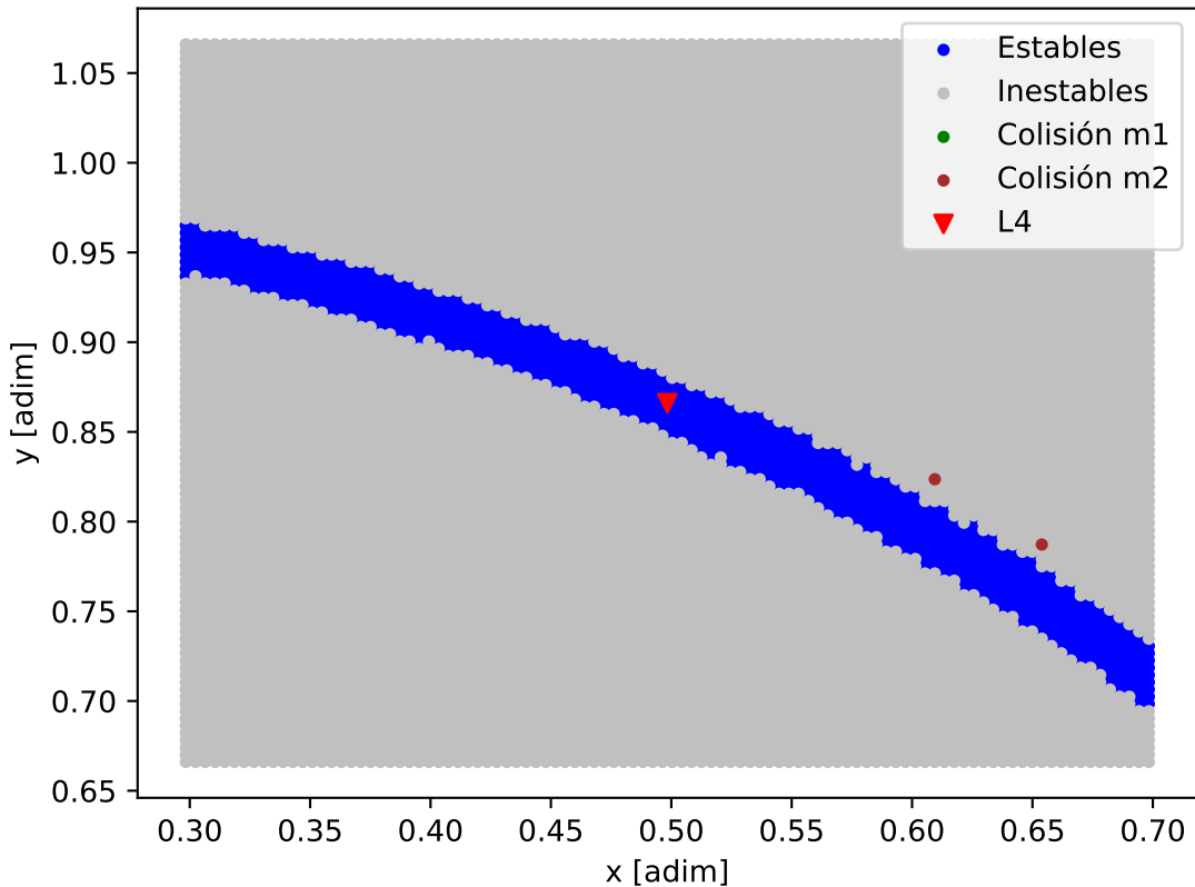
Mapa de estabilidad - HD_66428
