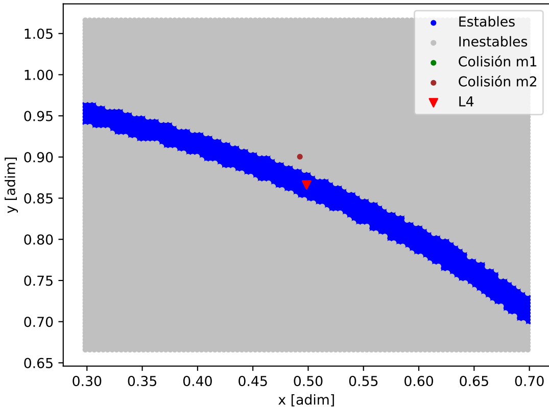
Mapa de estabilidad - HD_68988
