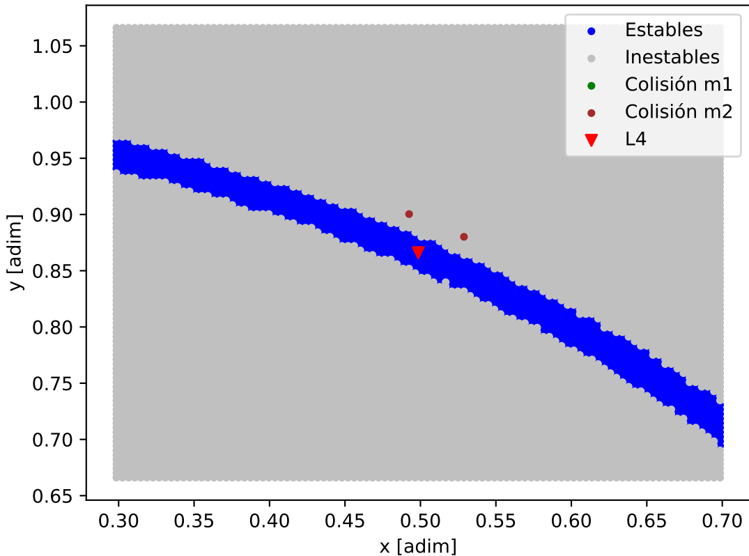
Mapa de estabilidad - HD_74156
