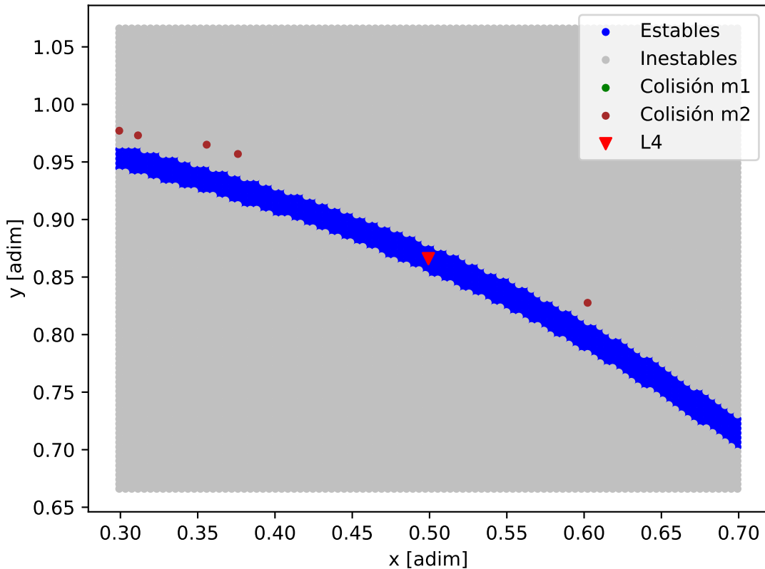
Mapa de estabilidad - HD_75784
