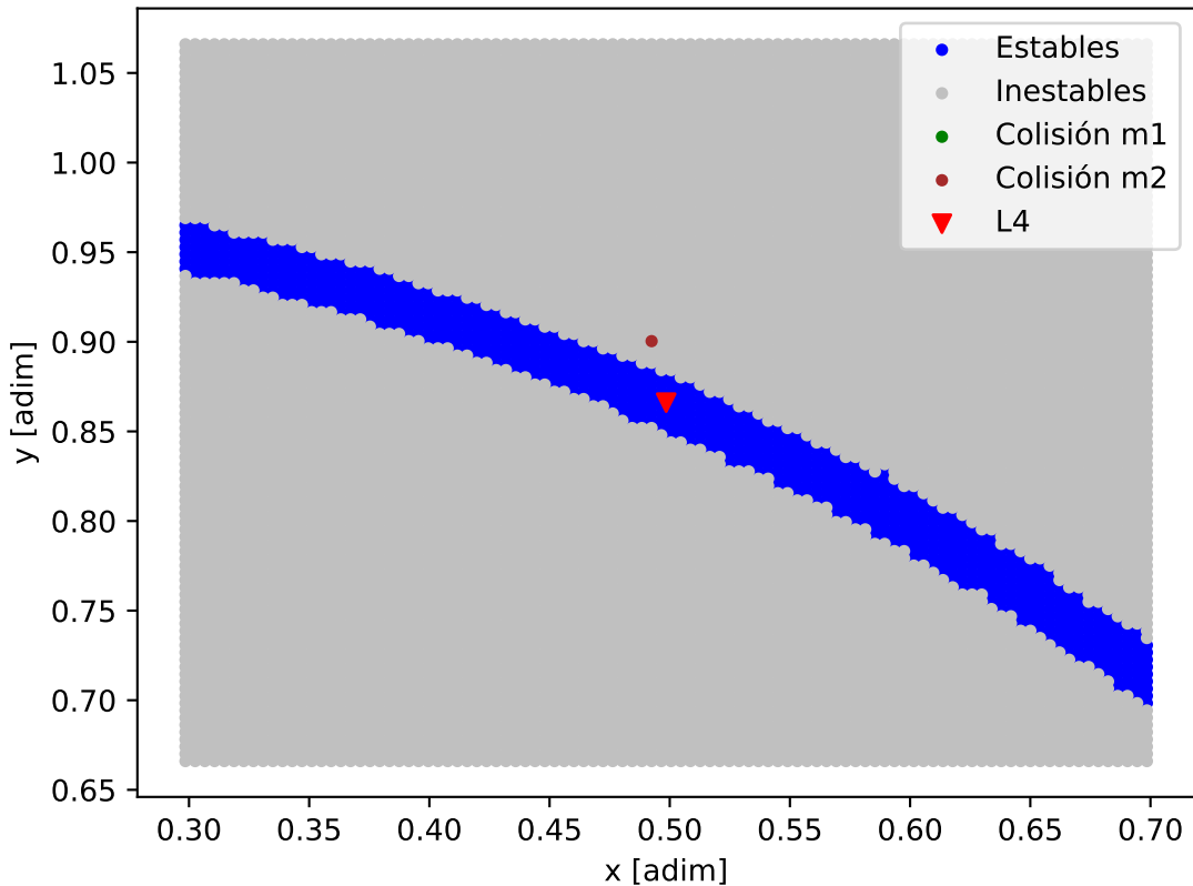
Mapa de estabilidad - HD_82943
