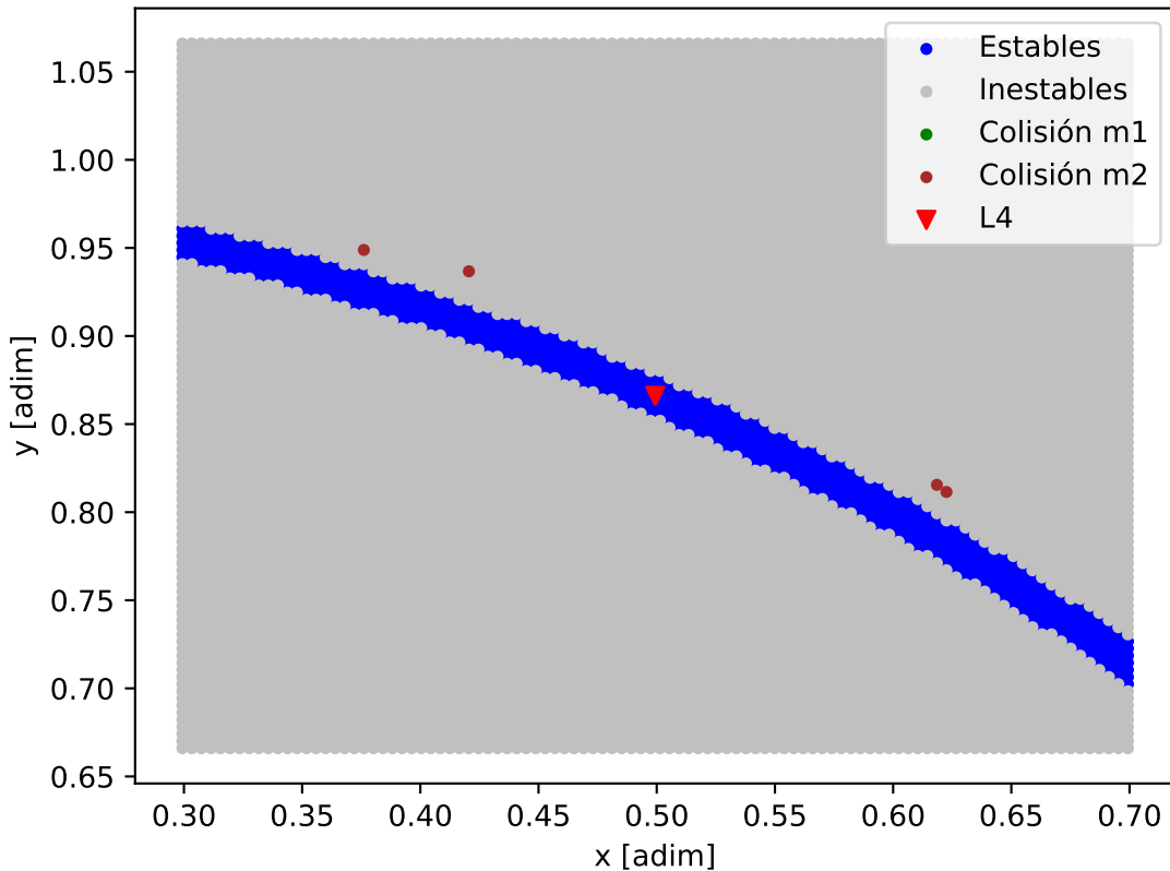
Mapa de estabilidad - HD_9446
