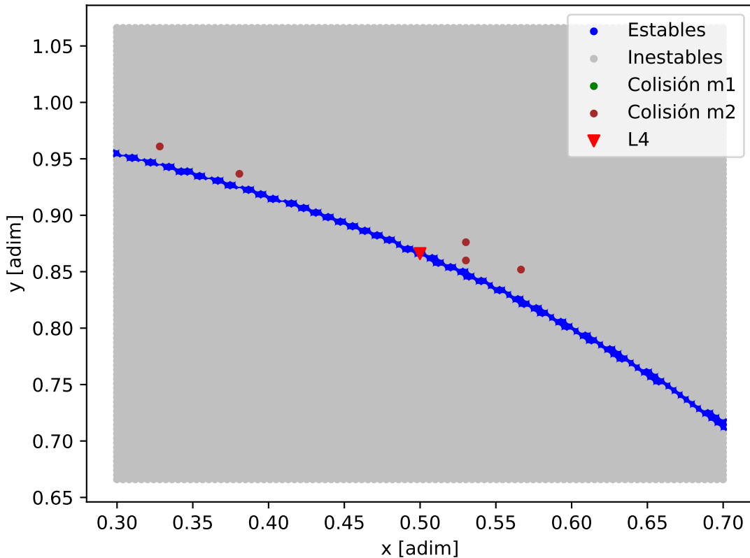
Mapa de estabilidad - K2-157
