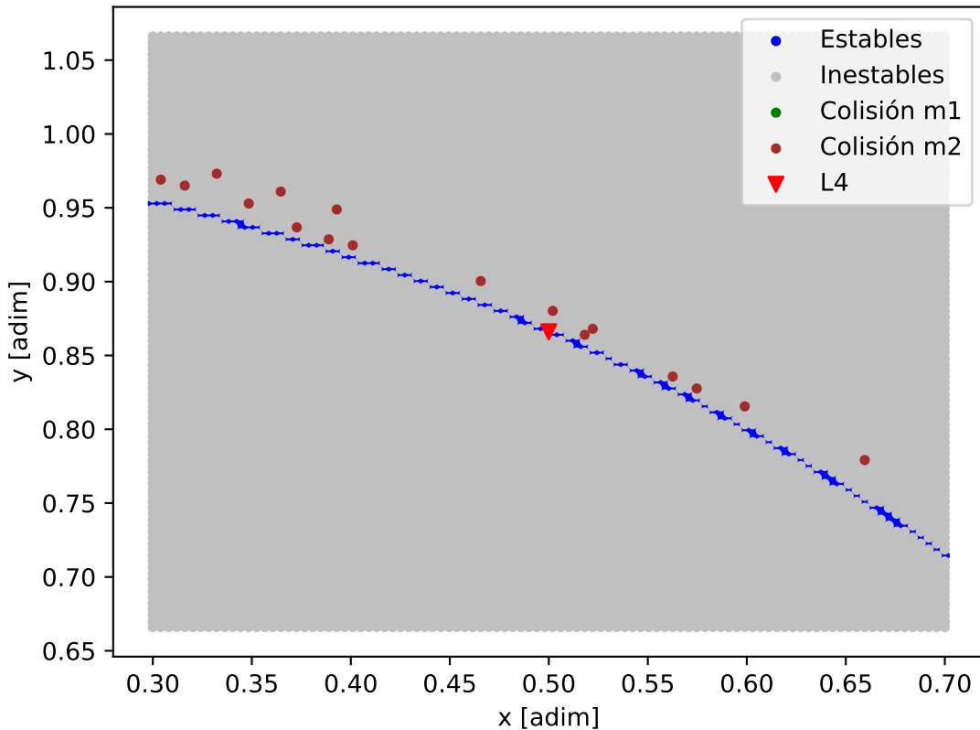
Mapa de estabilidad - K2-229
