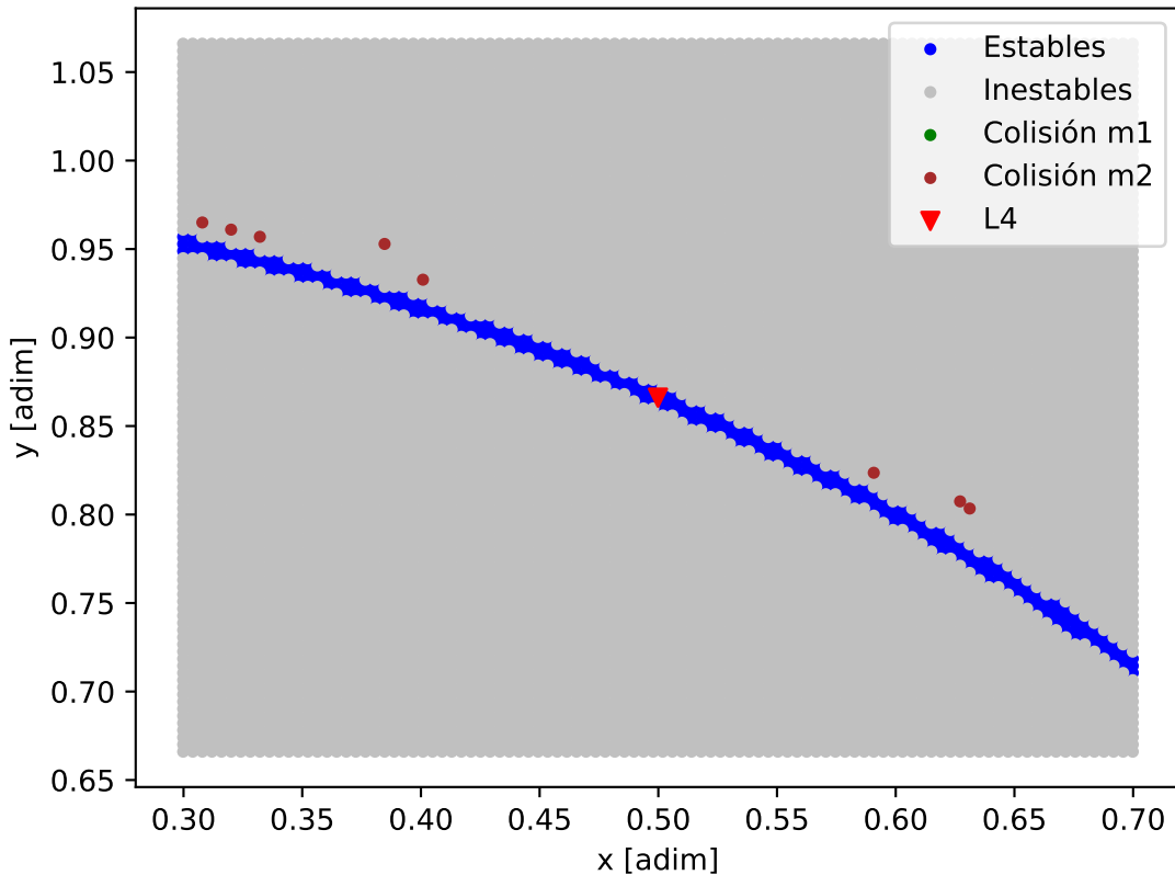
Mapa de estabilidad - Kepler-1513
