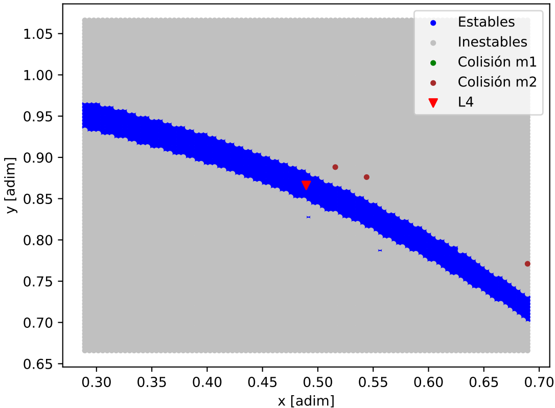
Mapa de estabilidad - OGLE-2019-BLG-0468L
