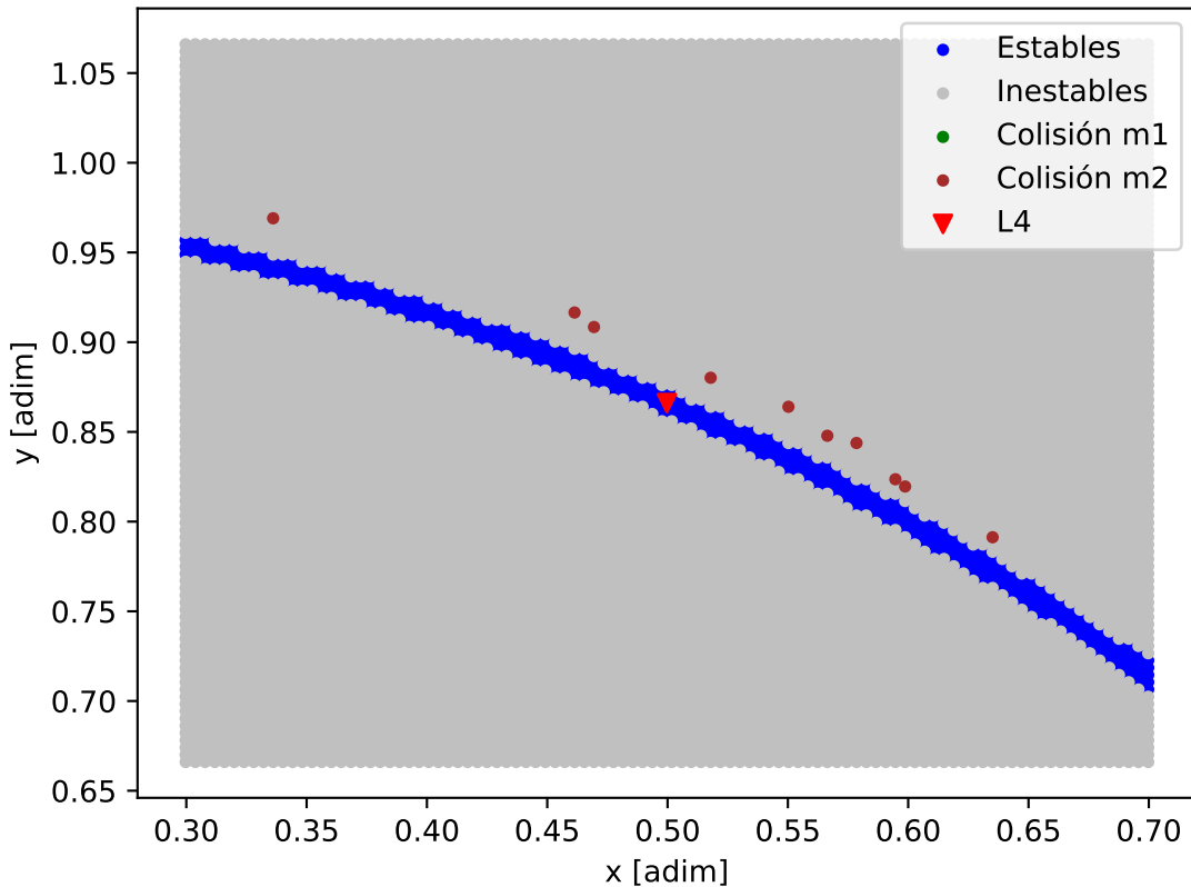
Mapa de estabilidad - TOI-1288
