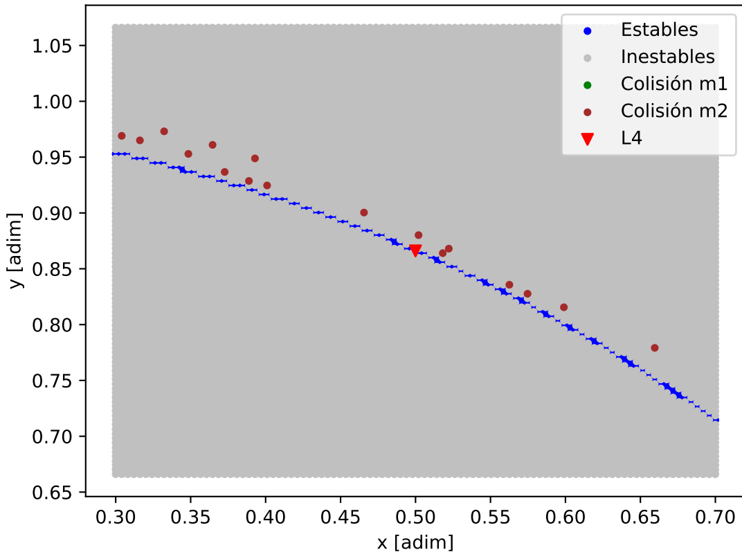
Mapa de estabilidad - TOI-421
