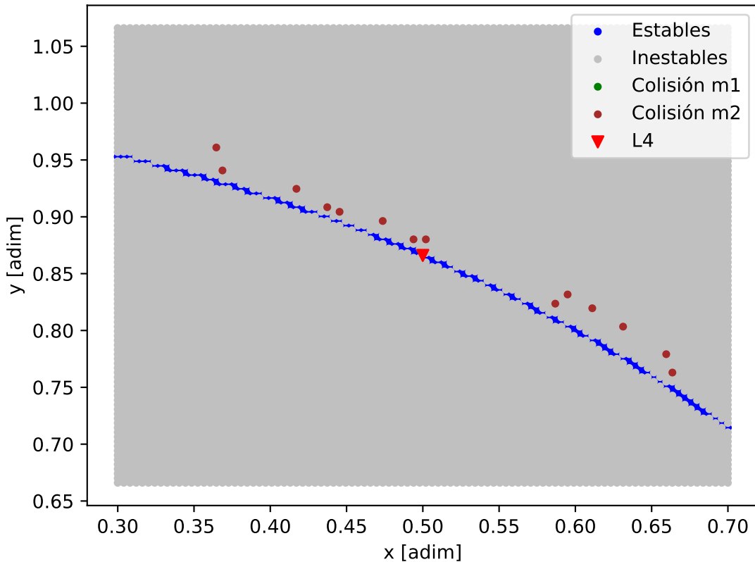
Mapa de estabilidad - TOI-451
