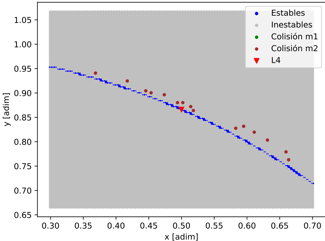
Mapa de estabilidad - TOI-5398
