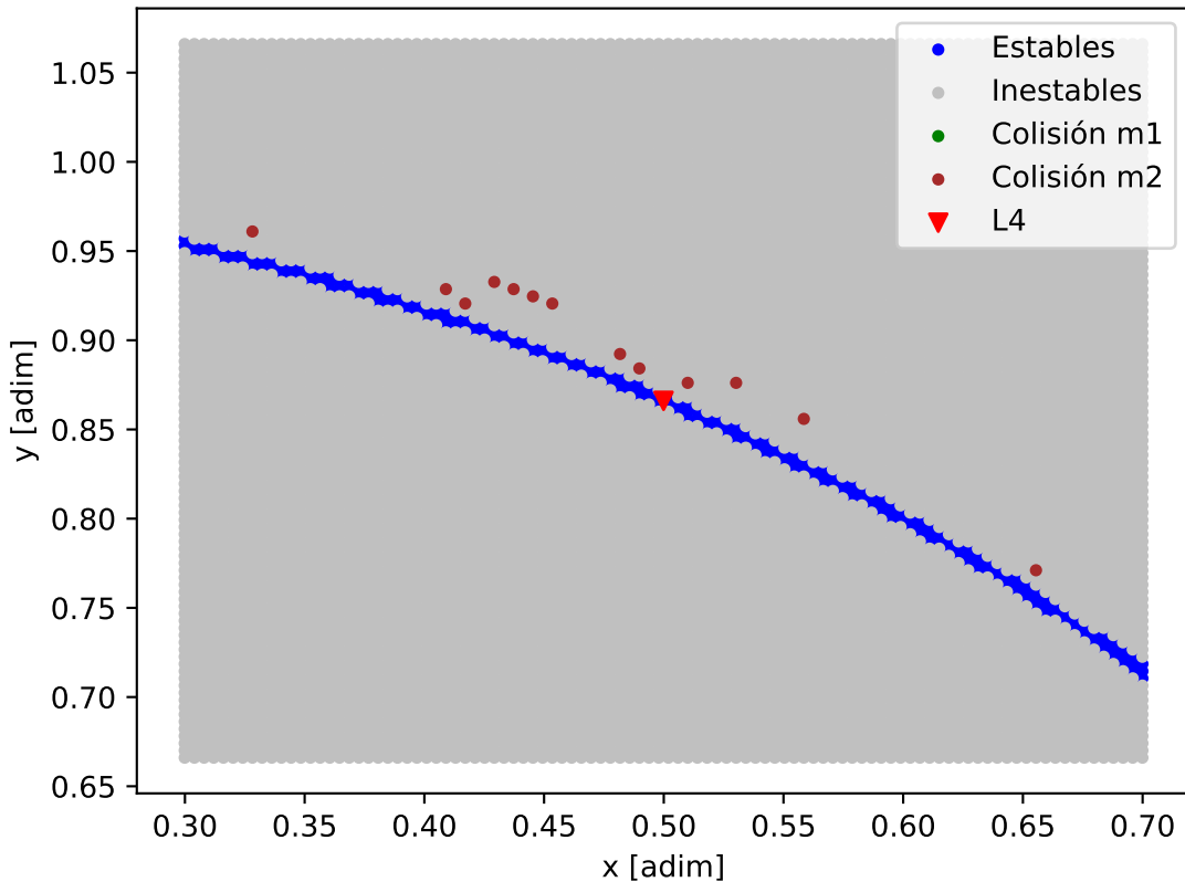
Mapa de estabilidad - CoRoT-24
