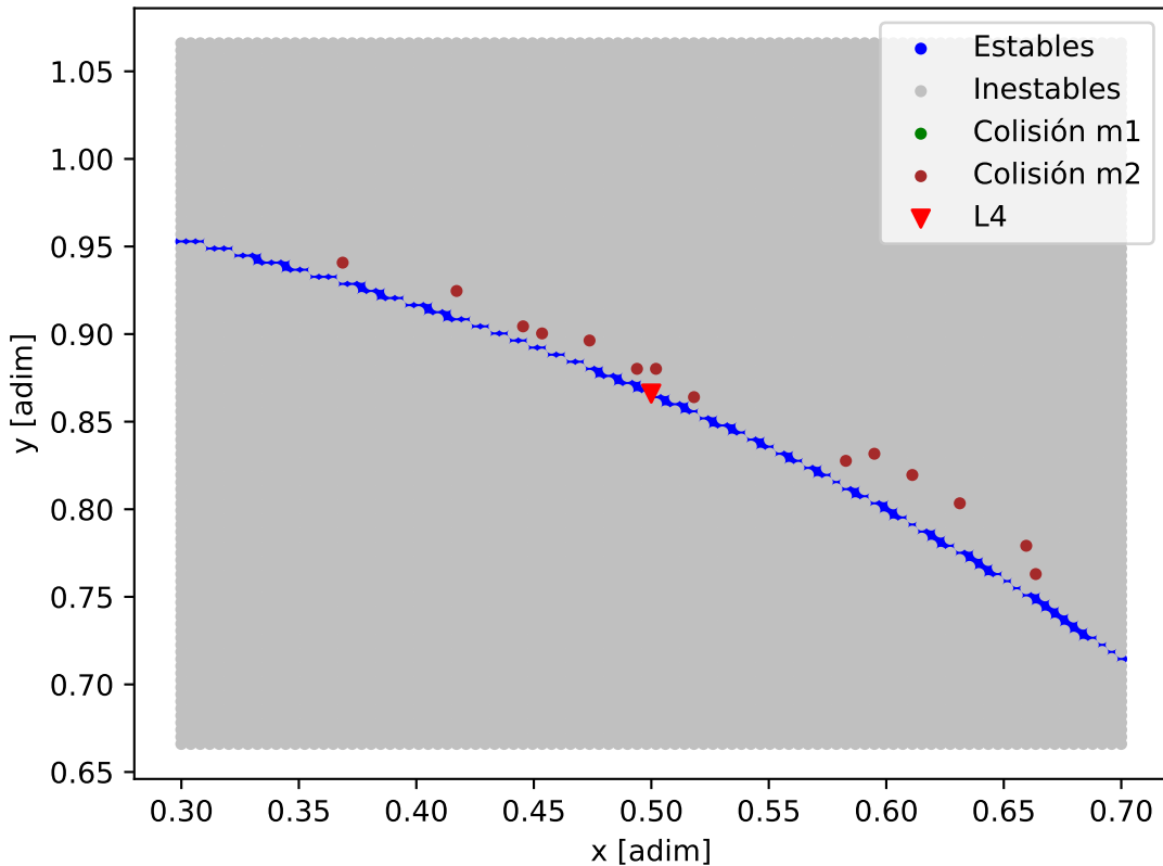
Mapa de estabilidad - EPIC_212737443
