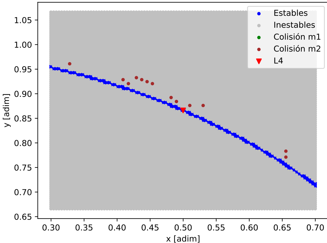
Mapa de estabilidad - GJ_143
