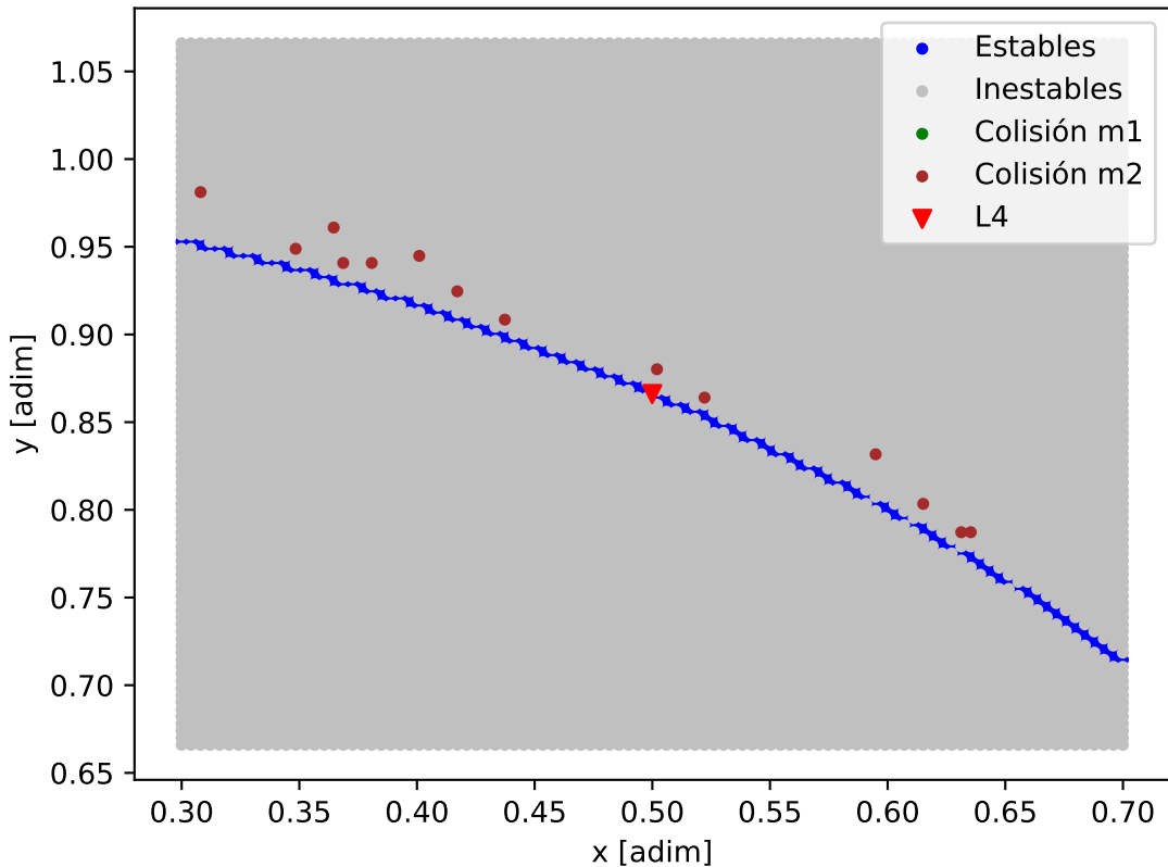
Mapa de estabilidad - HD_13808
