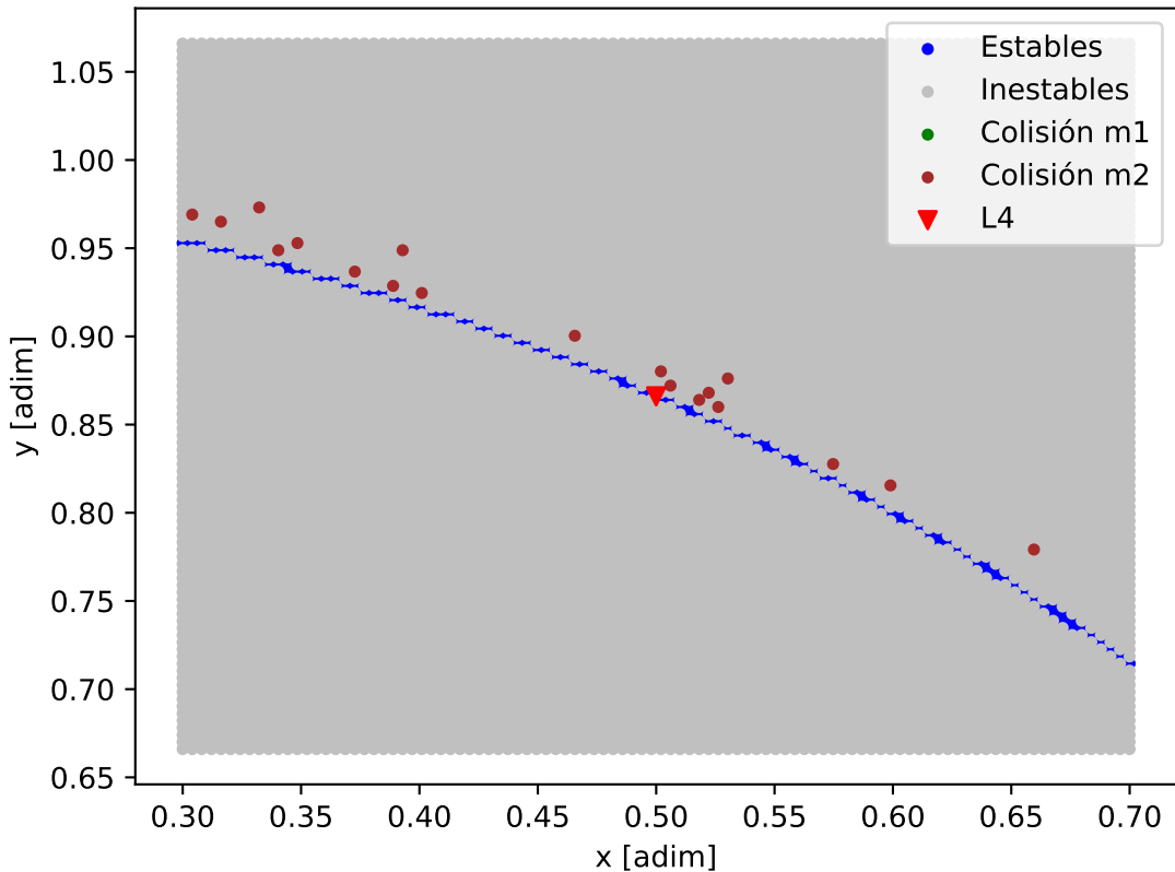
Mapa de estabilidad - HD_15337
